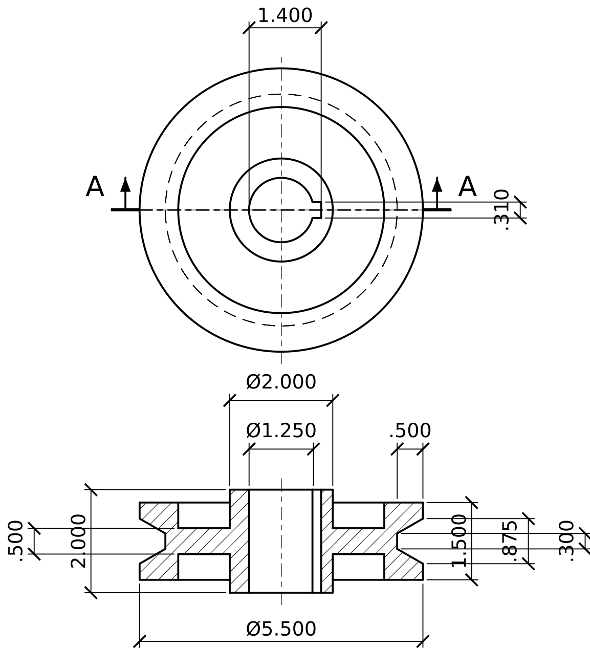
SECTION A-A
