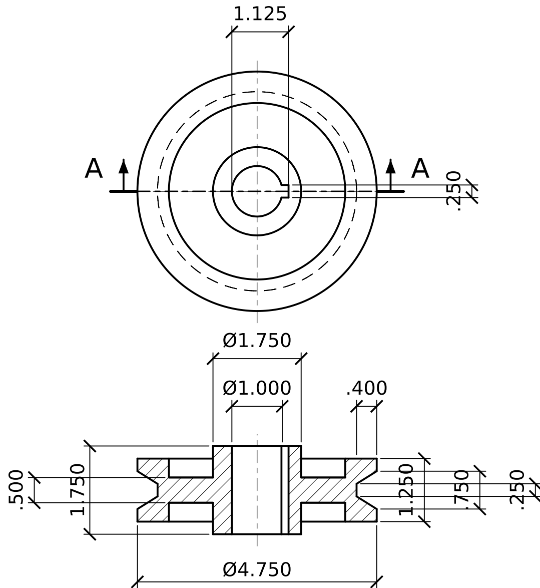
SECTION A-A
