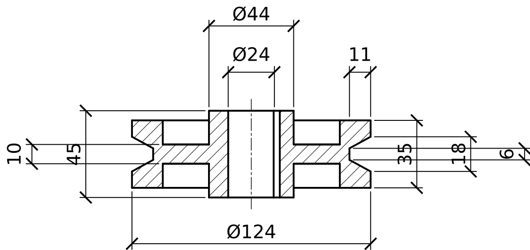
PRZEKRÓJ A-A
