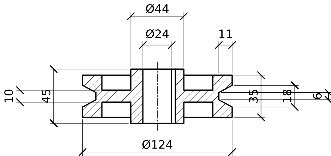
DOORSNEDE A-A
