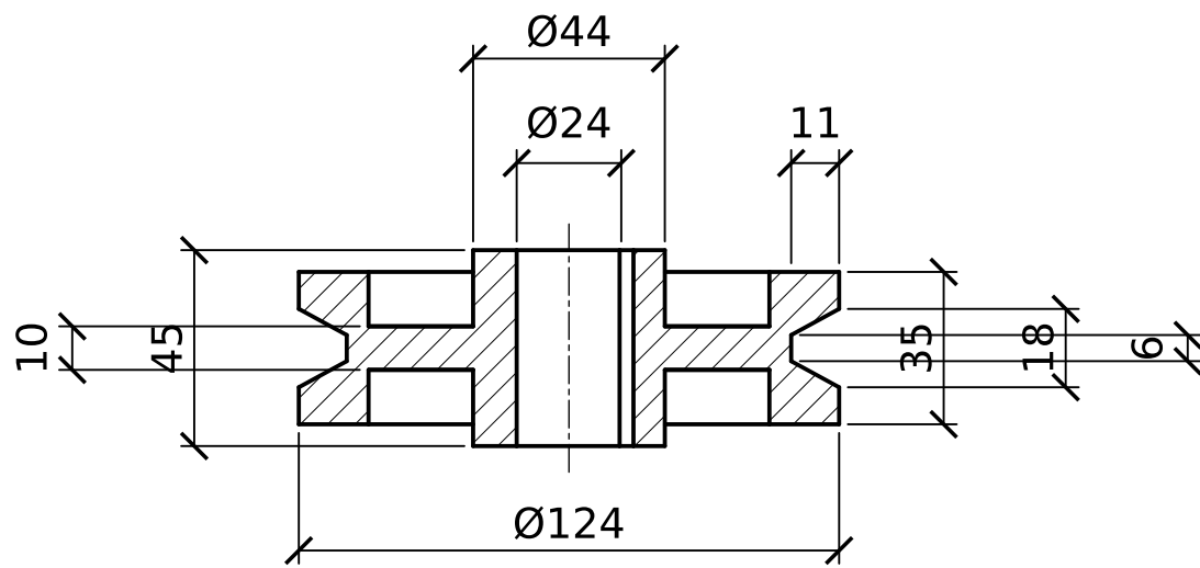
POTONGAN A-A
