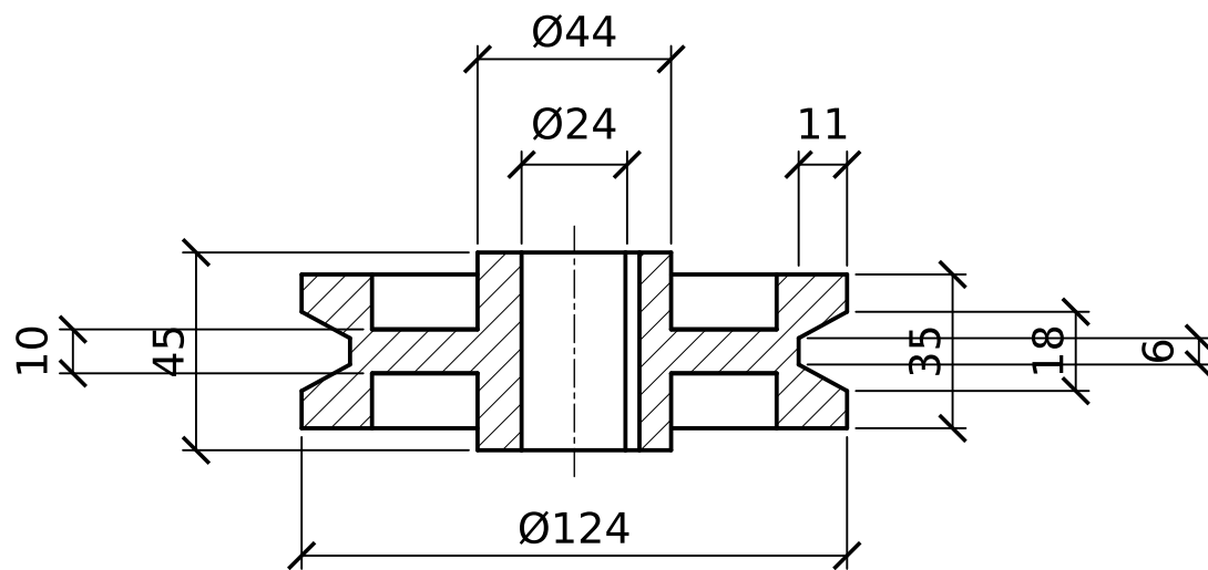
CORTE A-A
