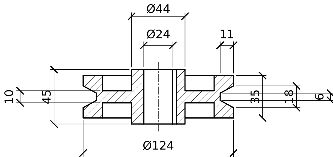
SCHNITT A-A
