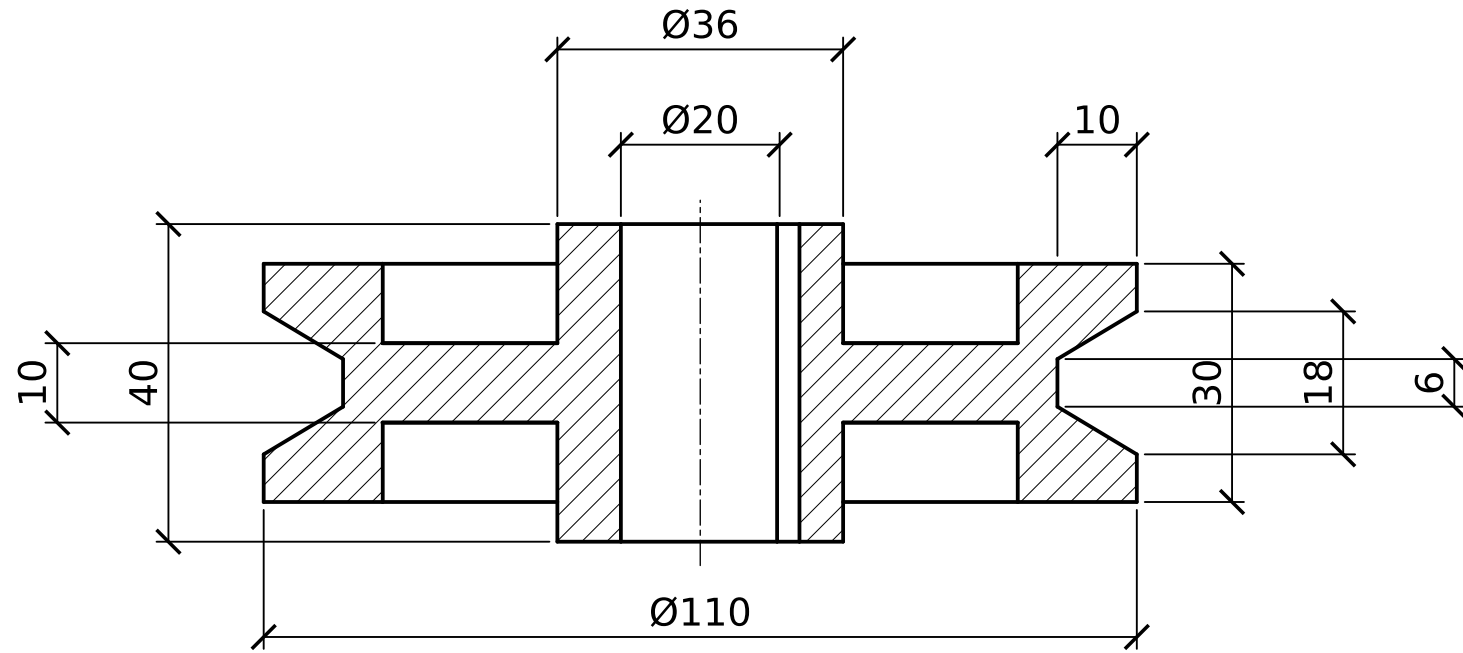
KESİT A-A
