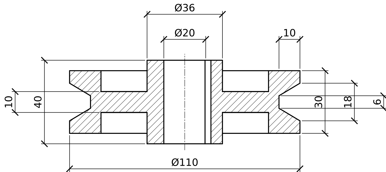
PRZEKRÓJ A-A
