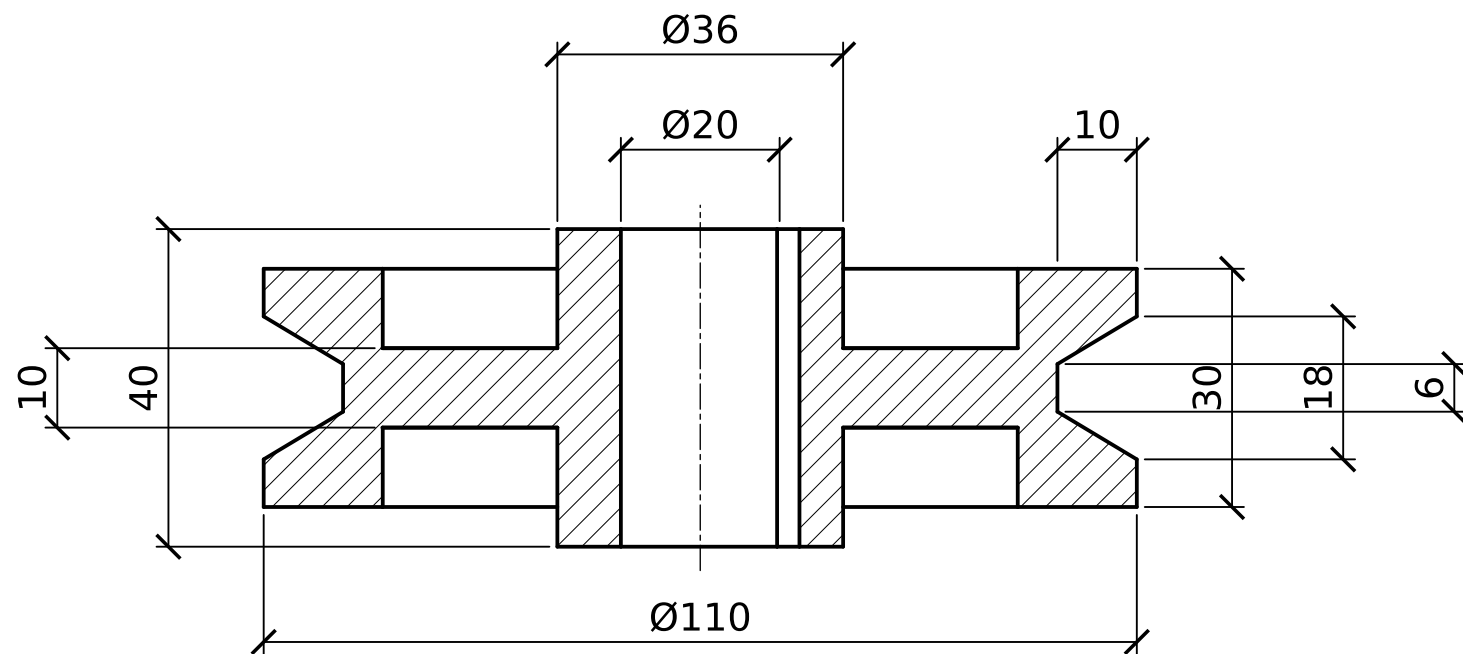
DOORSNEDE A-A
