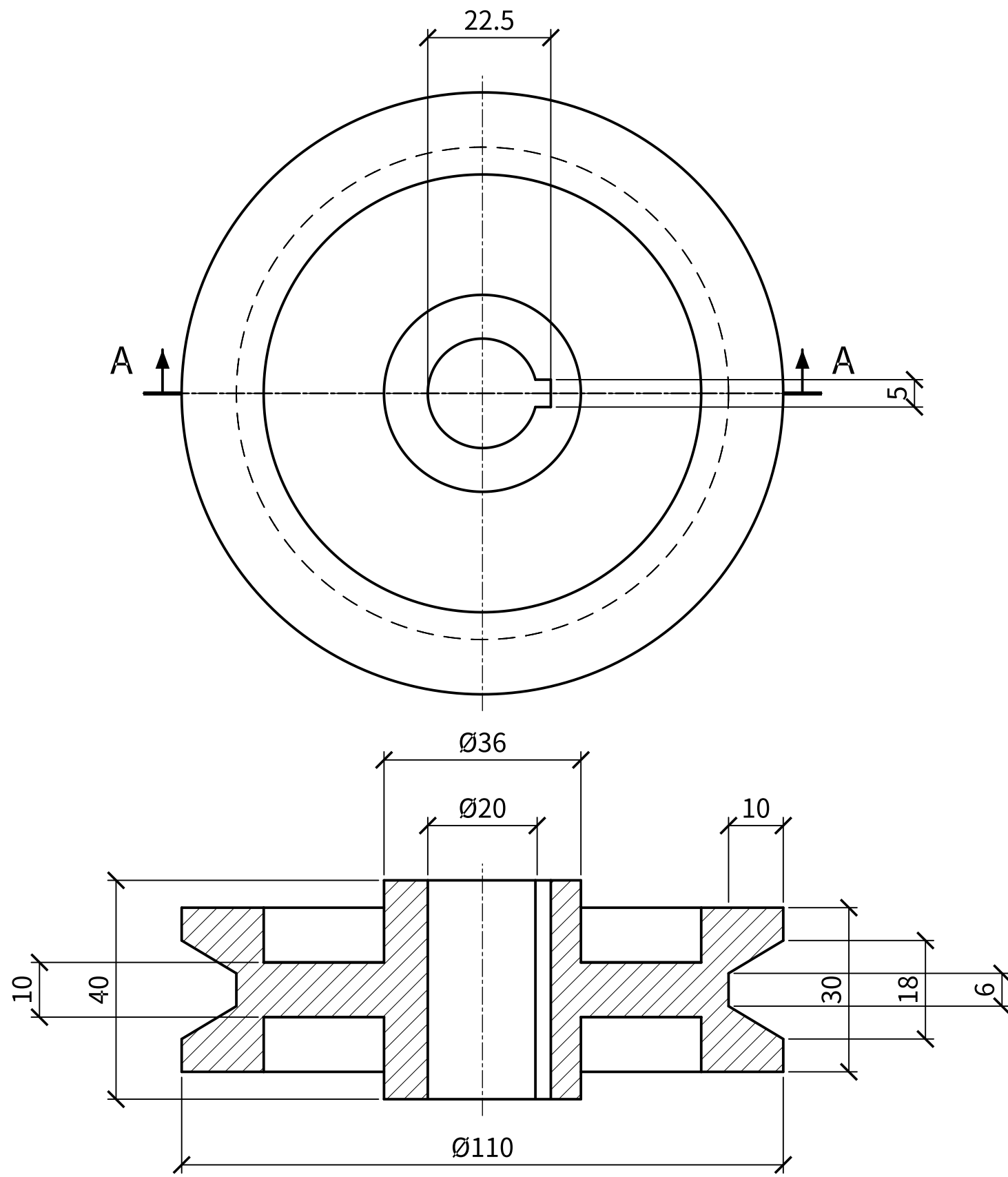
断面 A-A
