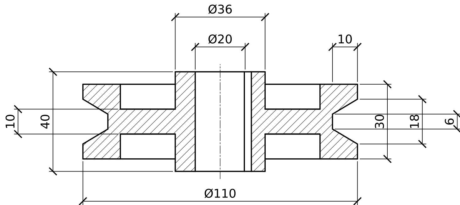
SEZIONE A-A
