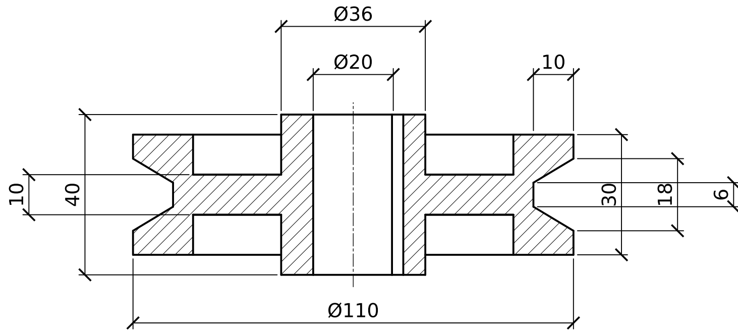
SECTION A-A
