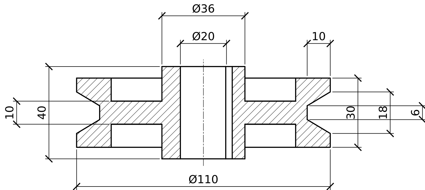
SCHNITT A-A
